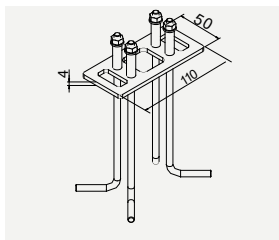
Art. 1907 3120062 Festejern Asker pullert Molde pullert
