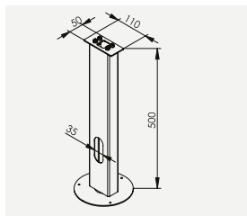
Art. 1908 3120063 Markfeste Asker pullert Molde pullert
