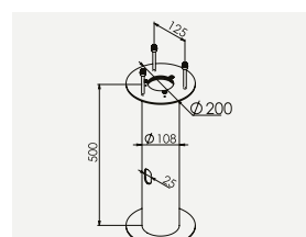
Art. 1231 3185546 Markfeste Stavanger Egersund
