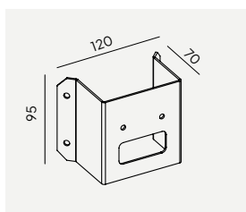
130GA 3104123 130B 3104124 Hjørnefeste Mandal
