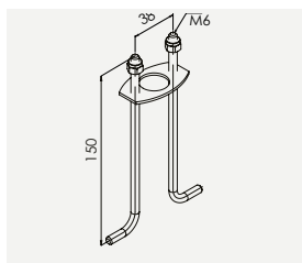
Art. 203 3102480 Festejern Borg
