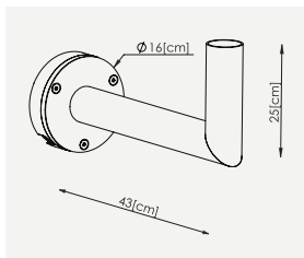
154AL 3185559 154GR 3185560 Veggfeste med arm Visby Nice Borg
