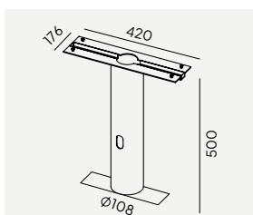
Art. 209 3104070 Markfeste Hellvik
