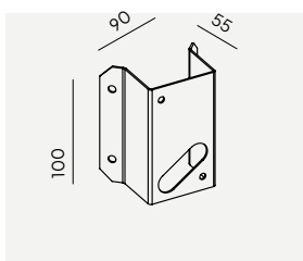
Art 131 Hjørnefeste Sandvik Art 1740, 1741, 1742, 5153
