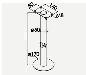
Art. 113 3101749 Markfeste Namsos
