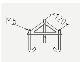
Art. 1128 Festejern Stockholm Art. 284, 285, 287 Medfølger alle modeller
