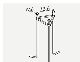
Art. 208 3101972 Festejern Arvika
