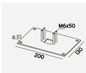
3081AL 3104110 3081GR 3104111 3081B 3104160 Fotplate Asker pullert Molde pullert
