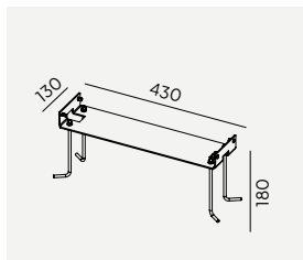
Art 2409 Festejern Hellvik
