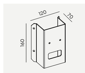
151GR 3102471 151AL 3102470 Hjørnebeslag Hitra
