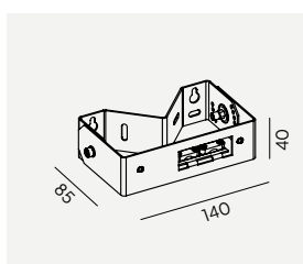
151GR 3102471 151AL 3102470 Hjørnebeslag Hitra
