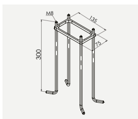
Art. 112 3101748 Festejern Namsos
