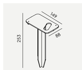
Art 1234 3185571 Jordspyd Sande
