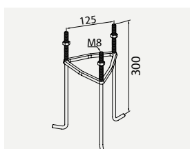
Art. 1230 3185545 Festejern Stavanger Egersund
