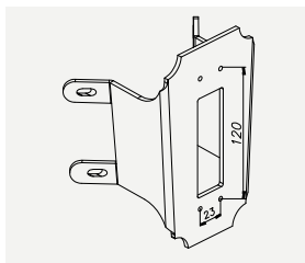
150B 3101731 150W 3183006 Hjørnebeslag Rimini
