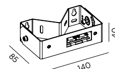
Art. 151GR Hjørnebeslag/Veggfeste (kan tiltes)
