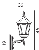
Art. 259 E27, 46W Halo max. Black, 259B White, 259W EEI: A+..D
