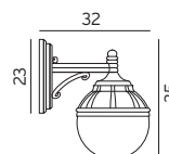
Art. 310 tinted globe. E27, 46W Halo max. Black, 310B White, 310W EEI: A+..D
