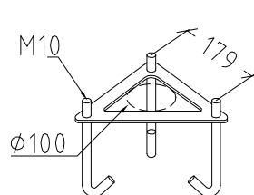
Art. 405ZZ Kit d'ancrage pour béton Koster Lofoten Lund Oslo Stockholm
