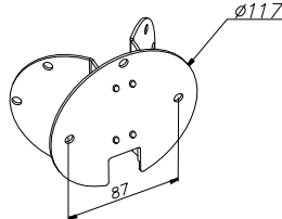
Art. 152 Pièce d'angle Bologna Chelsea Como Firenze London Modena
