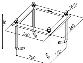
Art. 116ZZ Kit d'ancrage pour béton Asker (mât)
