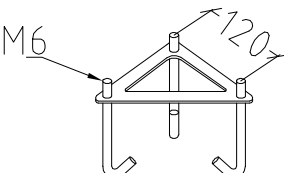
Art. 505ZZ Kit d'ancrage pour béton Narvik
