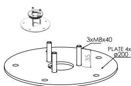
Art. 3080 Semelle pour bornes utilisant normalement 2052Z Alta Egersund Mini & Park Halmstad Kisa - Lillesand Lofoten Oppland Stockholm
