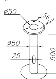
Art. 205ZZ Kit d'ancrage pour béton Alta Egersund Mini & Park Halmstad Kisa - Lillesand Lofoten Oppland Stockholm
