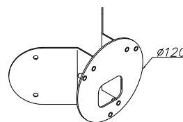
Art. 158 Pièce d'angle pour applique Koster
