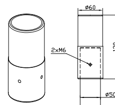
Art. 3061 Adaptateur pour mât Ø60 3061SV Noir 3061VI Blanc
