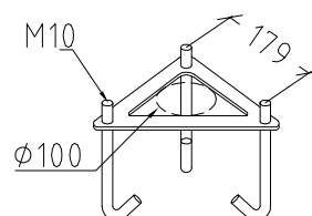
Art. 405ZZ Kit d'ancrage pour béton Koster Lofoten Lund Oslo Stockholm
