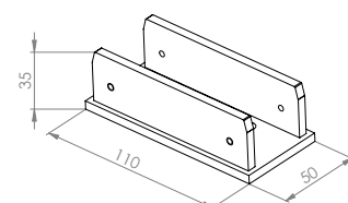
Art. 1906ZZ Fixation au sol en acier galvanisé Molde
