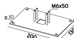
Art. 3050 Plaque murale gamme classique Bologna Como Firenze London Modena
