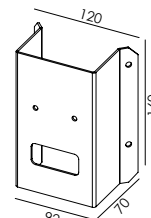
Art. 148 Pièce d'angle Sandvik Up & Down Art. 1730 Art. 1731 Art. 1732
