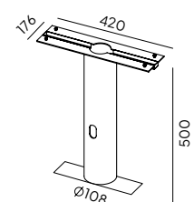
Art. 209 Markfeste 3104070
