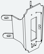
Art. 150 Hjørnebeslag Rimini
