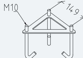
Art. 505 Festejern Narvik
