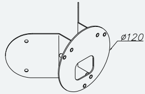
Art. 158 Hjørnebeslag Koster
