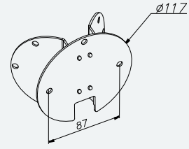
Art. 153 Hjørnebeslag Stockholm Oslo Lund Bergen Karlstad Vansbro Larvik
