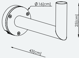
Art. 154 Veggfeste med arm Visby Nice Borg Hammerfest
