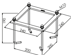
Art. 116 Ingjutningsfäste E 7748320 Asker stolpe
