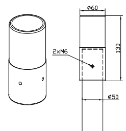
Art. 3070 Adapter för alla stolpar med \varnothing 50 mm ( \varnothing 50 - 60 mm) Alu, E 7703557 Grafit, E 7703558
