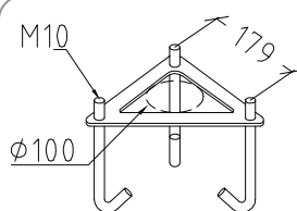
Art. 405 Ingjutningsfäste E 7722497 Stockholm Oslo Lund Rimini/Milano Koster Lofoten
