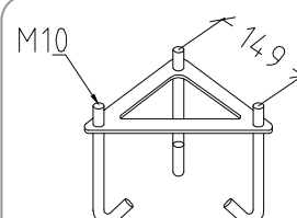
Art. 505 Ingjutningsfäste E 7748488 Narvik
