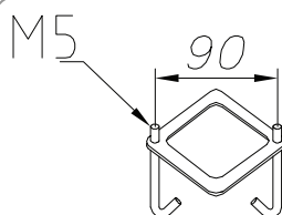
Art. 307 Ingjutningsfäste E 7722492 Chelsea Bologna London Modena Firenze
