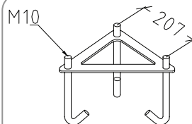
Art. 305 Ingjutningsfäste E 7722490 Chelsea Bologna London Modena Como Firenze
