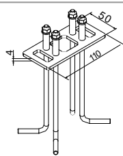
Art. 1907 Ingjutningsfäste E 7747458 Asker pollare Molde Hellvik
